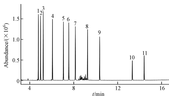
图 1 APs 和 BPA 的总离子流图(峰序号对应的化合物同表 1)
